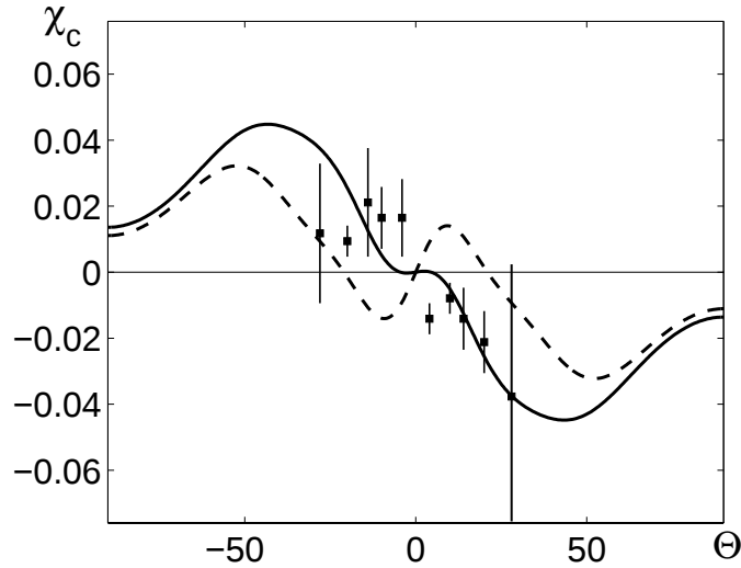
图 2.7: 发电机模型中与电流螺度相关参数 \langle \chi^c \rangle 随纬度变化与实际观测电流螺度 (黑色方块) 的对比。实线和虚线分别是两组发电机参数下与观测数据的拟合。
