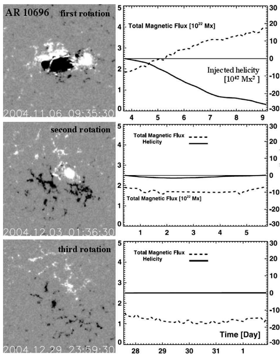
图 2.10: 活动区 AR10696 在三个太阳自转周的磁螺度积累, 左列是视向磁场的演化, 右列是相应的螺度积累 (实线) 和磁通量 (虚线) 随时间的演化。其中左轴标注是磁通量, 右轴标注是磁螺度。
