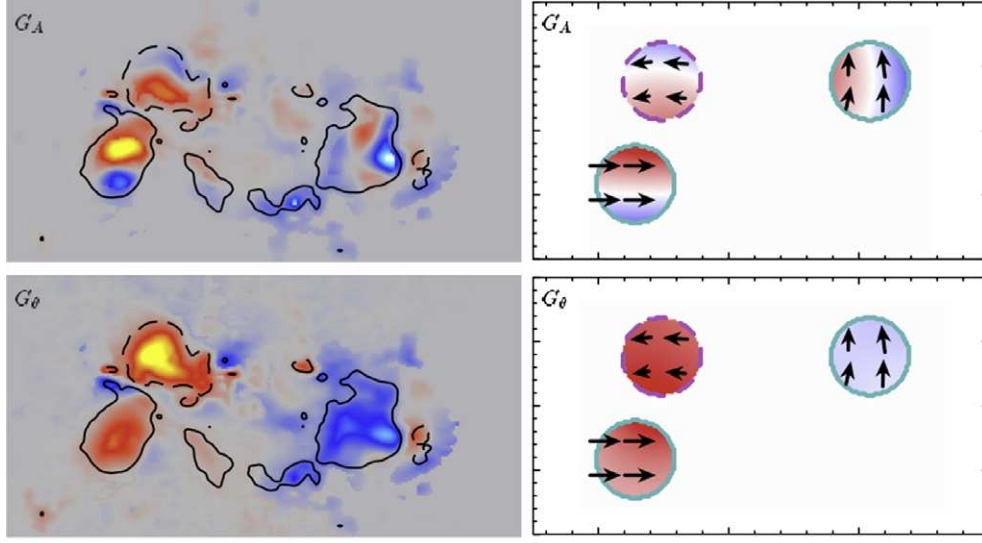
图 2.5: 两种方法计算得到的活动区 AR9182 的螺度传输率分布图的比较。左列是实际计算的结果, 右列是建立活动区模型的结果。第一行是 G_A 的分布图, 第二行是 G_\theta 的分布图。可以明显看到在 G_A 图中同一极性中存在有相反的螺度传输率; 而在 G_\theta 图中是不存在相反极性。
