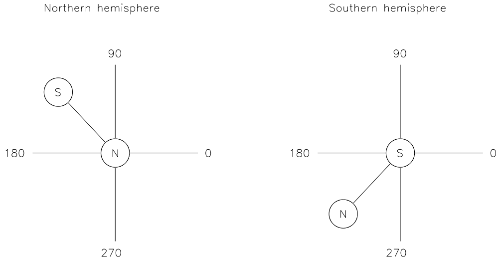
图 3.3: 本文使用的磁倾角 (Ta) 的图示。左图 (右图) 是描述南 (北) 半球。Ta 的取值范围是 0^\circ \sim 360^\circ 。
