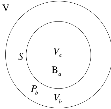
图 2.3: 相对螺度的传输示意图。
