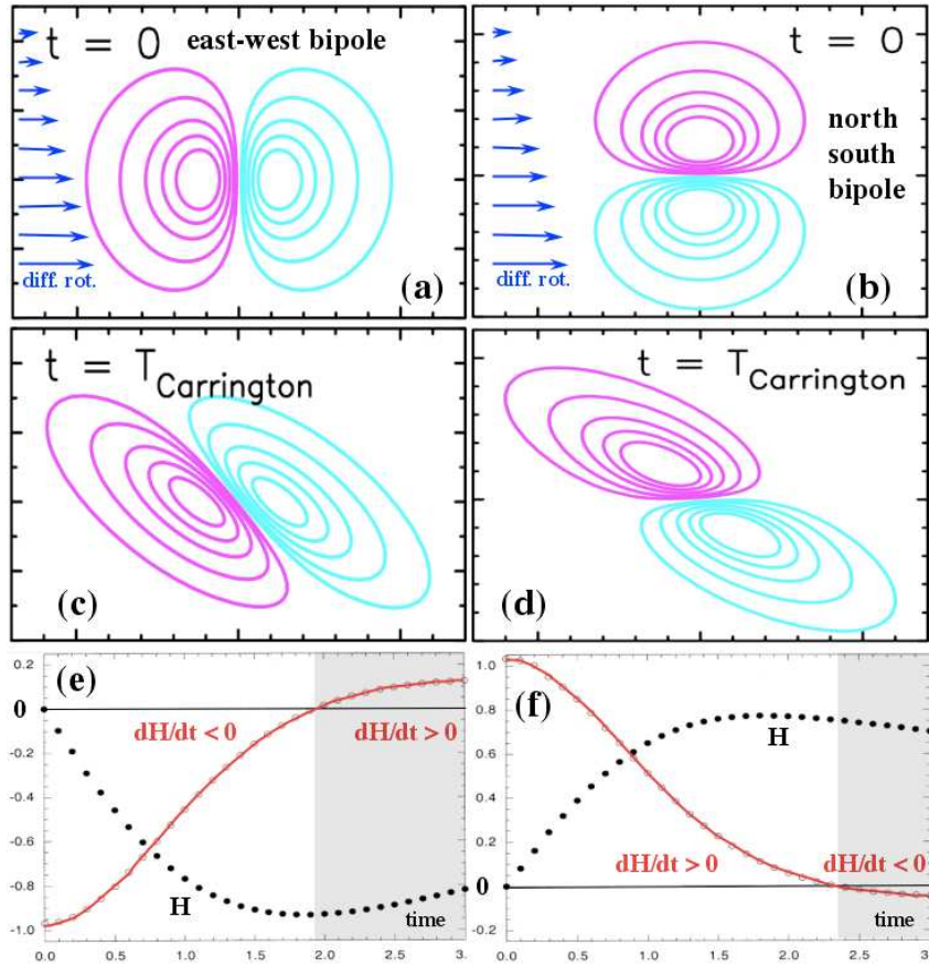
图 2.13: 北半球偶极活动区在较差自传下的螺度传输。左右两列两图分别对应着两种初始状态下的演化。 t=0 对应着初始磁场位形 (a 和 b); t=T 对应着最终的磁场位形 (c 和 d)。e 和 f 分别对应着两种情况下的螺度传输率和积累螺度可以看到同样在北半球, 同样的较差自传速度分布情况下两者的螺度传输符号是相反的。
