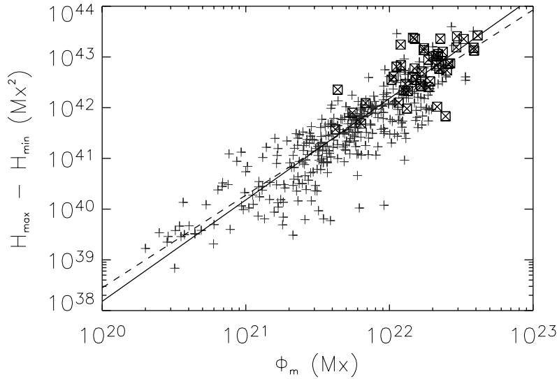
图 2.11: 积累螺度和磁通量之间的关系。
